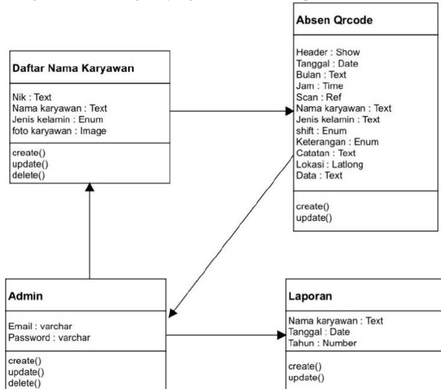
Gambar 9. Class Diagram Sistem Informasi Presensi
